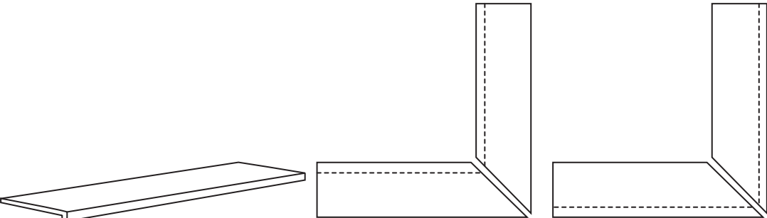
PELDAÑO ANGULAR ANTISLIP 120 x 32/3 (G 72) 48" x 12,5"/1" 60 x 32/3 (G 73) 23,6" x 12,5"/1"
