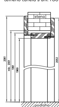
Vertikálna časť nastaviteľného tunela s uhl. T80
