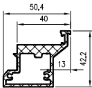
DRE profil pre dovnútra otvá- ratelné reverzné falcové dvere
