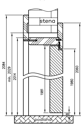
Vertikálny prierez ORO
