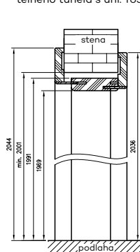
Vertikálna časť nastaviteľného tunela s uhl. T63
